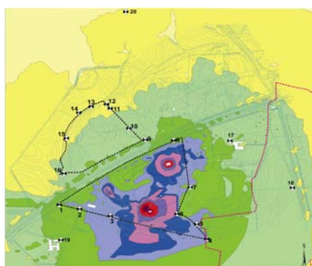
Modélisation bruit
